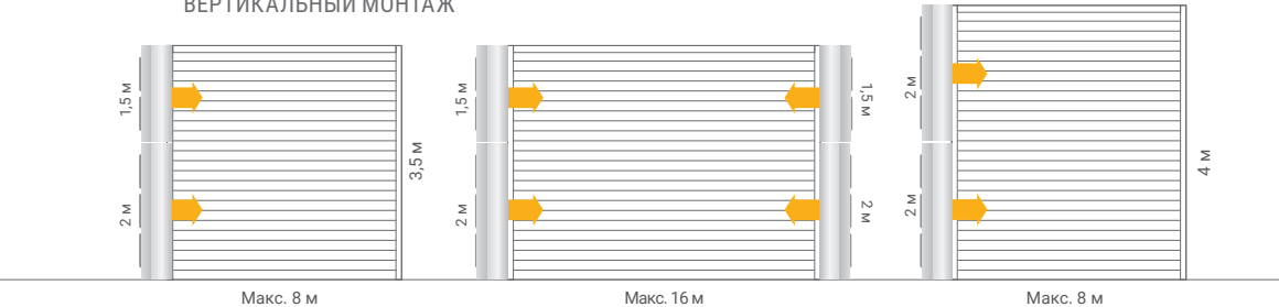
ВЕРТИКАЛЬНЫЙ МОНТАЖ
