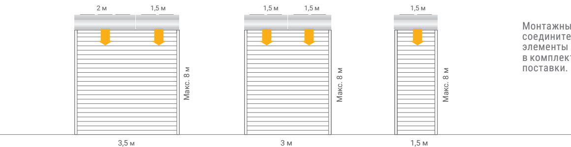
ВЕРТИКАЛЬНЫЙ МОНТАЖ
